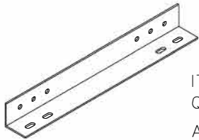
ITEM # 2 QTY: 4 Angle, Incline, 25.5" Long
